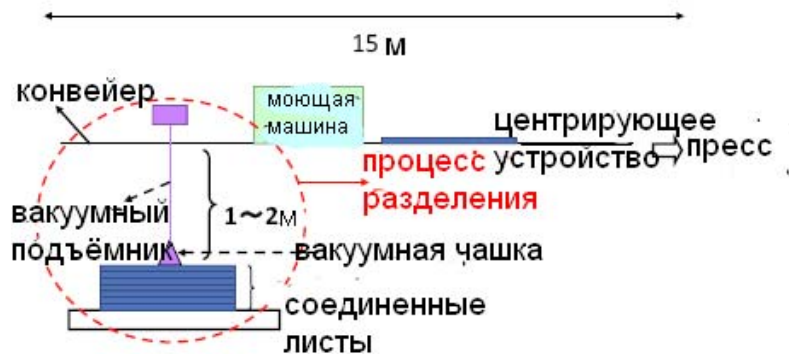
Рисунок 3: Макет подачи листов алюминия.
